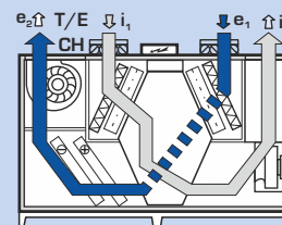
Ventilation uden varmegenvinding (via bypass)
